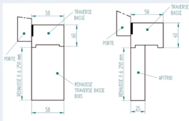
Modèle en applique
