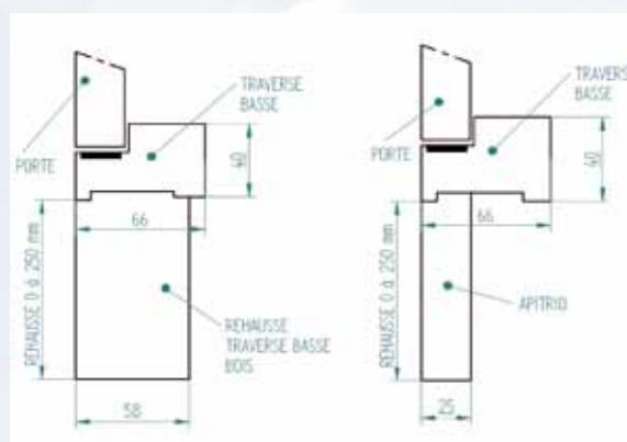
Modèle en feuillure
